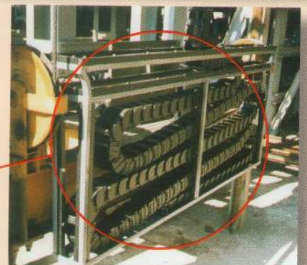
Специальное исполнение энергетических цепей, так называемое «складной метр» для горизонтальной прокладки привода
